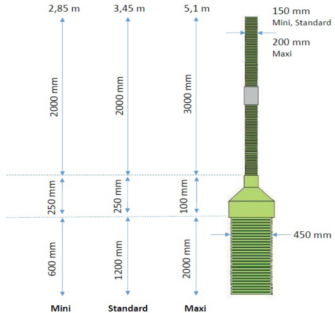
Abb. 1. Ausführungen der Polycool Säulen
